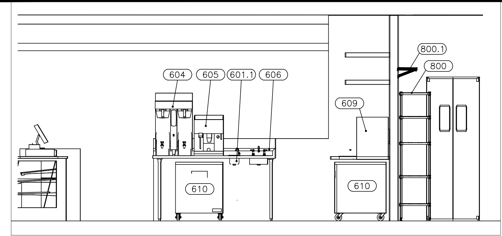
8 BARISTA ELEVATION K-401 SCALE: 3/8" = 1'-0"
