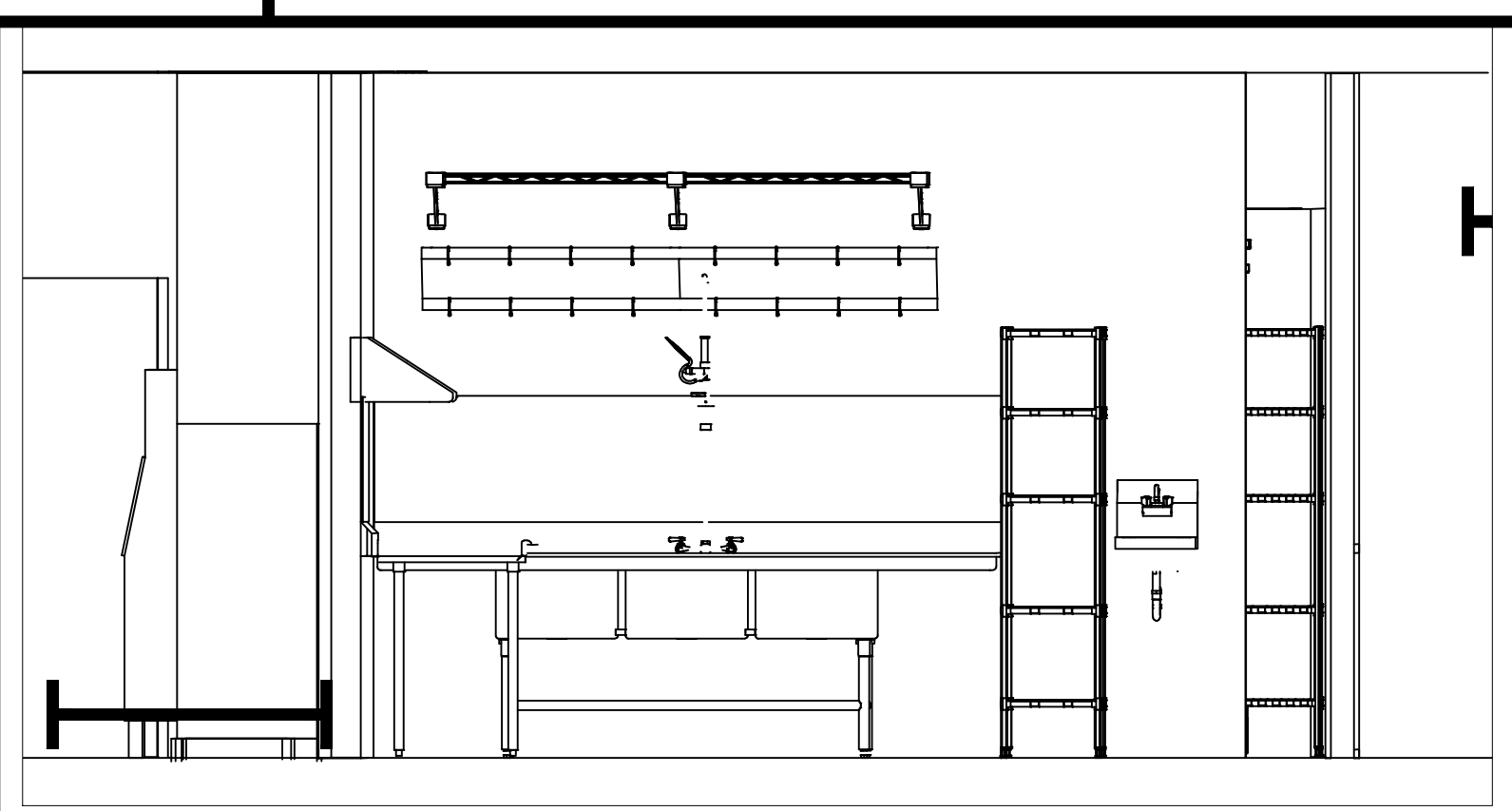
13 3-BOWL SINK ELEVATION K-401 SCALE: 3/8" = 1'-0"
