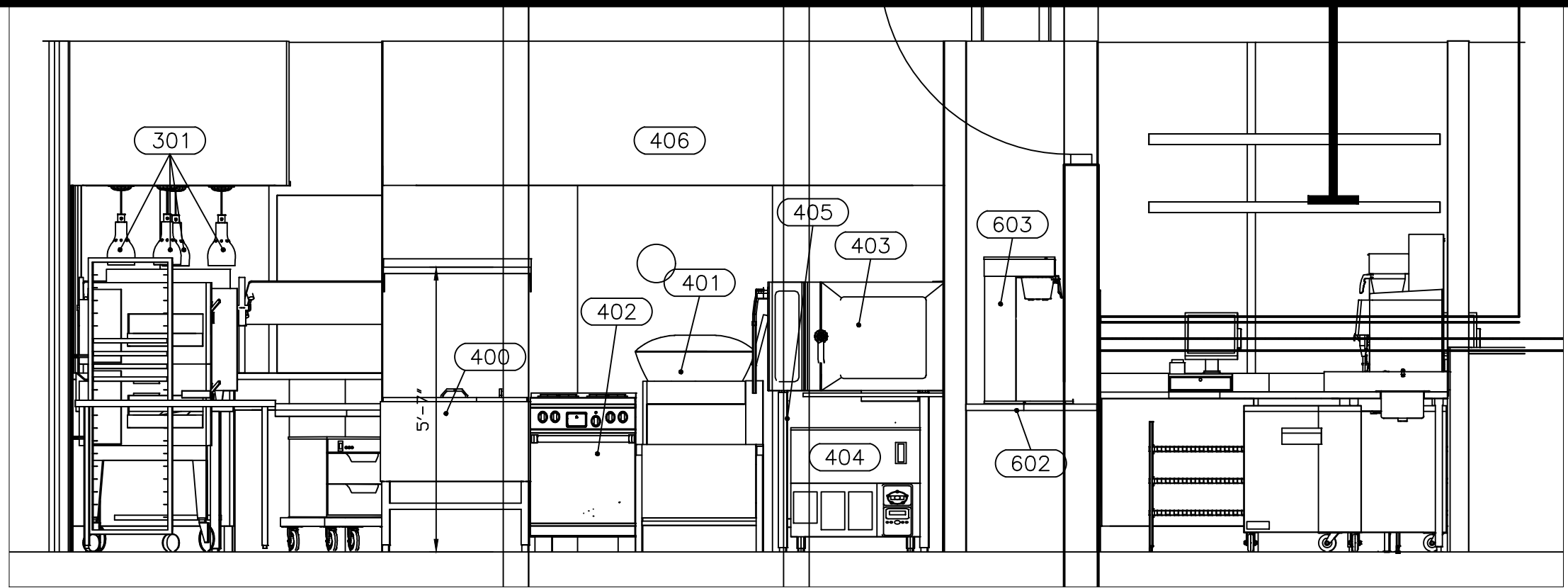
5 HAND SINK ELEVATION K-401 SCALE: 3/8" = 1'-0"
