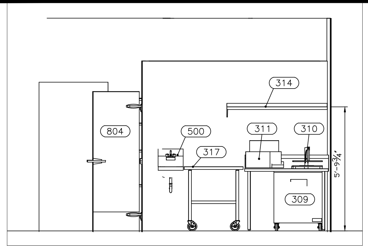
4 HAND SINK ELEVATION K-401 SCALE: 3/8" = 1'-0"
